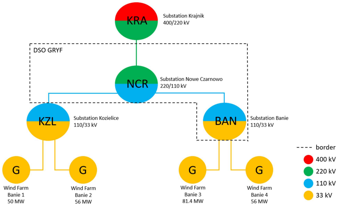
Rysunek 1 Schemat blokowy OSD GRYF wraz z infrastrukturą sąsiadującą
